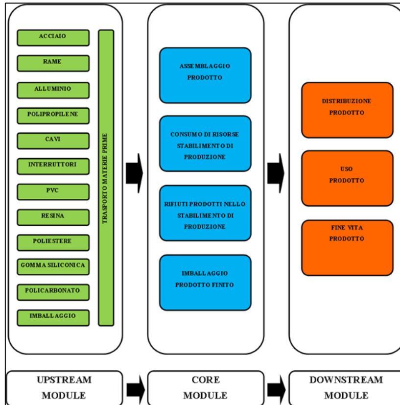
Figura 2: Diagramma di flusso dei confini del sistema
