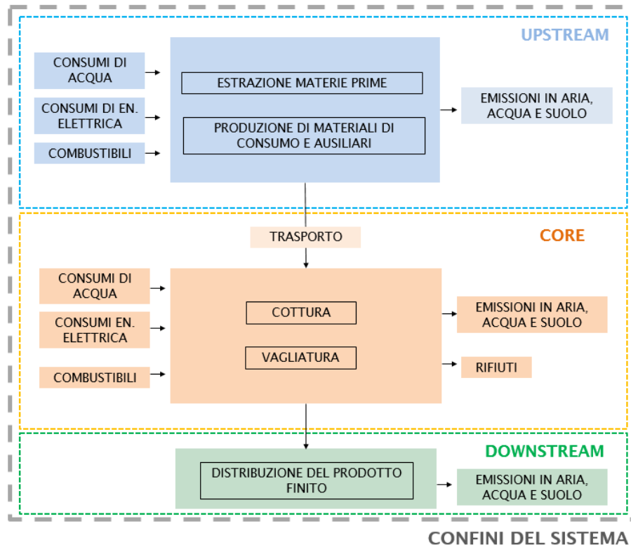
Figura 2 – Flowchart della produzione di calce viva calcica e confini del sistema.
