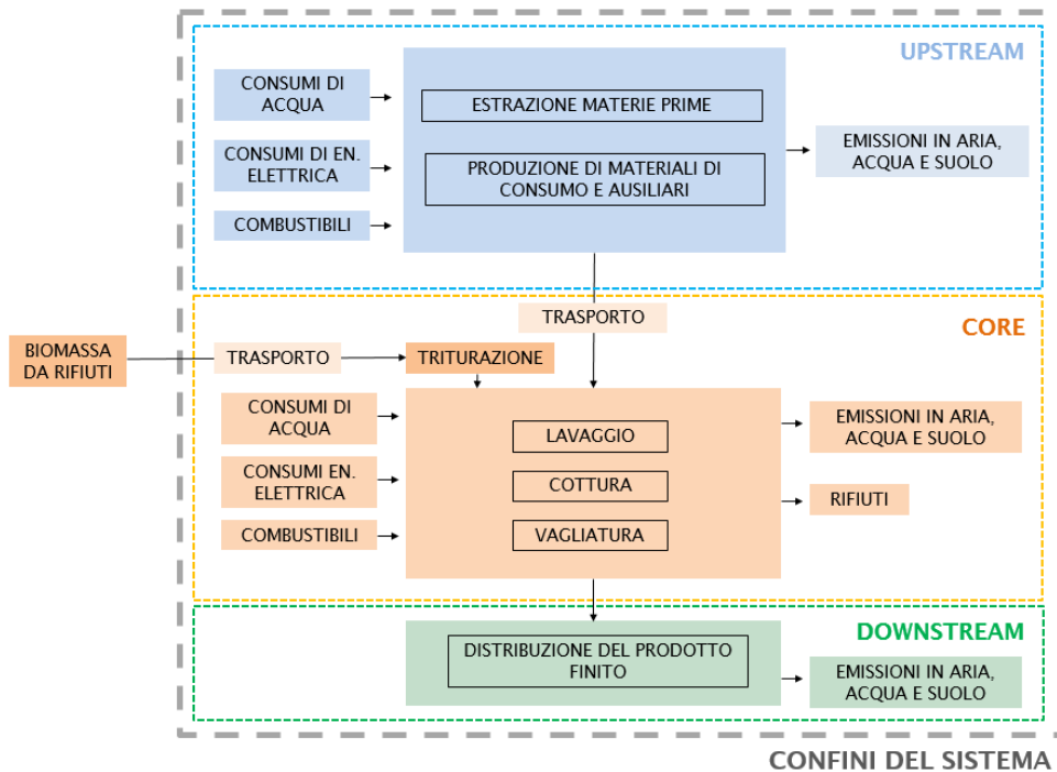
Figura 2 – Flowchart della produzione di calce viva calcica e confini del sistema.
